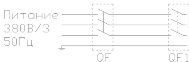
Рис.1. Схема подключения изделия к электросети
