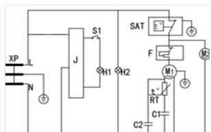
SD-206/336/416 AMLC/AML XP - штгелсель ашасы; SAT - Термостат; S1 - артқы жарық қосқышы; F - қорғаныс релесі; J - қуат қалқаны; M1 - Компрессор; H1 - ішкі подсветка; H2 - қуат индикаторы; M2 - салқындату желдеткіші; RT - Стартер; C1 - іске қосу сыйымдылығы (жүзеге асыру кезінде); C2 - пайдалану сыйымдылығы (жүзеге асыру кезінде)
