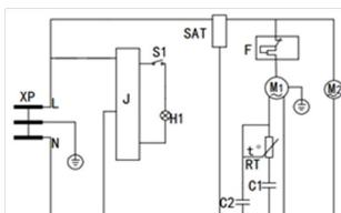
SD-206/336/416AELC/AEL XP - штгелсель ашасы; SAT - Термостат; S1 - артқы жарық қосқышы; F - қорғаныс релесі; J - қуат қалқаны; M1 - Компрессор; H1 - ішкі подсветка; M2 - желдеткіш салқындату; RT - Стартер; C1 - іске қосу сыйымдылығы (жүзеге асыру кезінде); C2 - пайдалану сыйымдылығы (жүзеге асыру кезінде)
