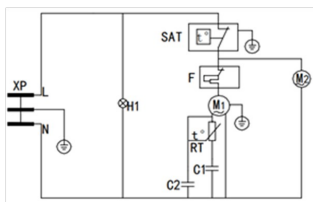
SD-206/336/416 AMC/AM XP - штгелсель ашасы; SAT - Термостат; F - қорғаныс релесі; M1 - Компрессор; H1 - қуат индикаторы; M2 - салқындату желдеткіші; RT - Стартер; C1 - іске қосу сыйымдылығы (жүзеге асыру кезінде); C2 - пайдалану сыйымдылығы (жүзеге асыру кезінде)
