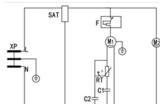
SD-206/336/416AEC/AE XP - штгелсель ашасы; SAT - Термостат; F - қорғаныс релесі; M1 - Компрессор; M2 - салқындату желдеткіші; RT - Стартер; C1 - іске қосу сыйымдылығы (жүзеге асыру кезінде); C2 - пайдалану сыйымдылығы (жүзеге асыру кезінде)
