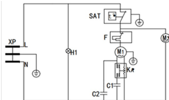
SD-516AMC/AM XP - штгелсель ашасы; SAT - Термостат; F - қорғаныс релесі; H1 - қуат индикаторы; M1 - Компрессор; M2 - желдеткіш салқындату; KA - Стартер; C1 - іске қосу сыйымдылығы (жүзеге асыру кезінде); C2 - пайдалану сыйымдылығы (жүзеге асыру кезінде)
