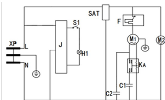
SD-516AELC/AEL XP - Штгелсель ашасы; SAT – Термостат; S1 - Артқы жарық қосқышы; F - қорғаныс релесі; J - қорек қалқаны; M1 - Компрессор; KA - Стартер; H1 - ішкі подсветка; M2 – Салқындату желдеткіші; C1 - іске қосу сыйымдылығы (жүзеге асыру кезінде); C2 - Пайдалану сыйымдылығы (жүзеге асыру кезінде)
