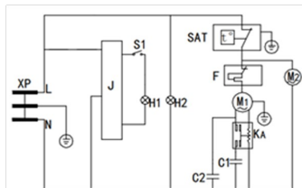
SD-516AMLC/AML XP - Штгелсель ашасы; SAT - Термостат; J-қорек қалқаны; S1 - артқы жарық қосқышы; F - қорғаныс релесі; M1-Компрессор; H1 - ішкі подсветка; H2-қуат индикаторы; M2-салқындату желдеткіші; KA-Стартер; C1 - іске қосу сыйымдылығы (жүзеге асыру кезінде); C2-пайдалану сыйымдылығы (жүзеге асыру кезінде)
