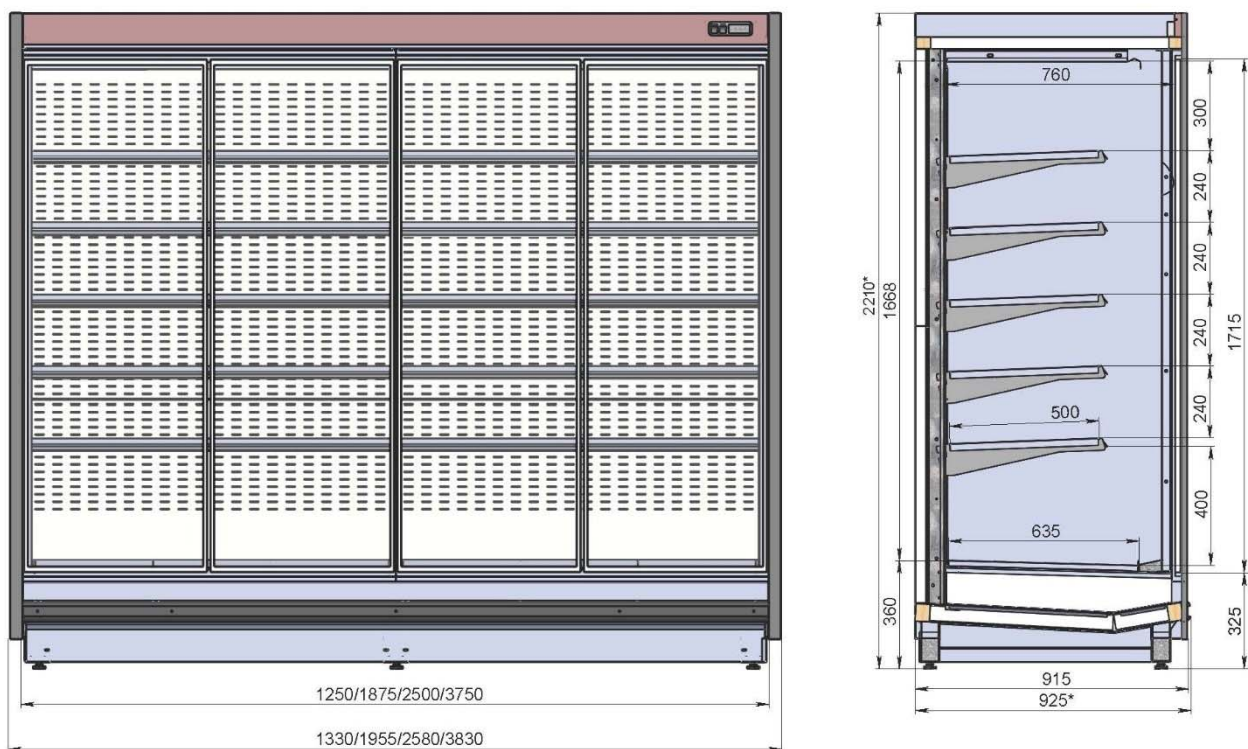
Рис.1. Внешний вид и основные размеры Sonata с дверьми
