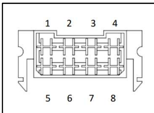
Распиновка шлейфа
